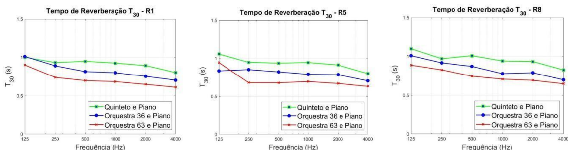
Figura 7: Resultados das simulações do TR nos receptores 1, 5 e 8, nos três cenários, com a Fonte B.
