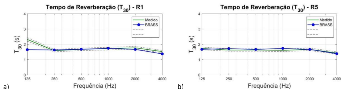
Figura 4: Resultados das simulações de TR x medições de TR (sala com janelas abertas).
