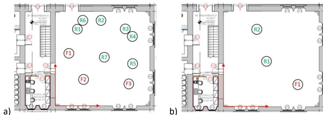
Figura 1: Planta baixa da sala de ensaios e pontos de medição, janelas fechadas (a) e abertas (b).
