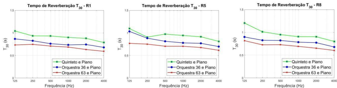
Figura 6: Resultados das simulações do TR nos receptores 1, 5 e 8, nos três cenários, com a Fonte A.
