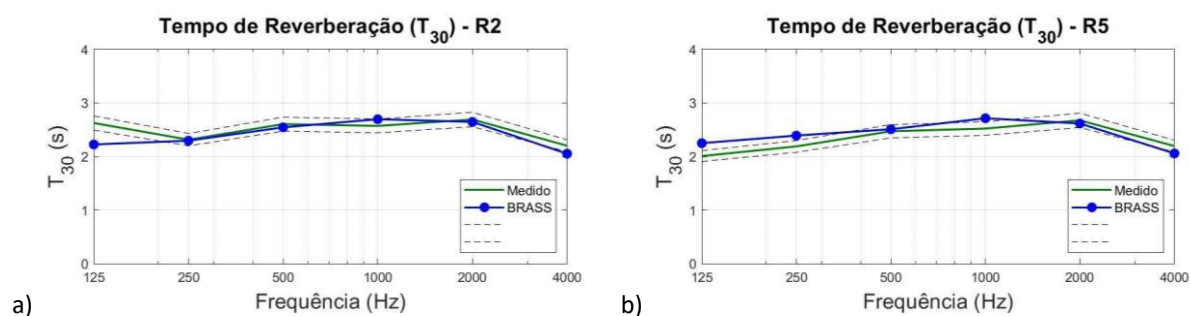
Figura 3: Resultados das simulações de TR x medições de TR (sala com janelas fechadas).
